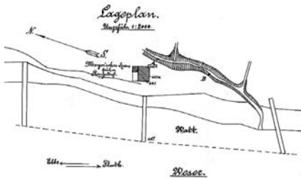
Lageplan der Pegelstation Farge am Fährhaus aus dem Jahr 1903. Der dreiteilige Lattenpegel ist mit A, B und C gekennzeichnet.
